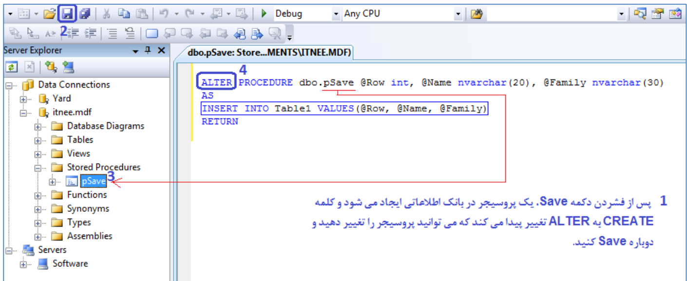
شکل ۹ - ایجاد پروسیجرهای ذخیره شده
