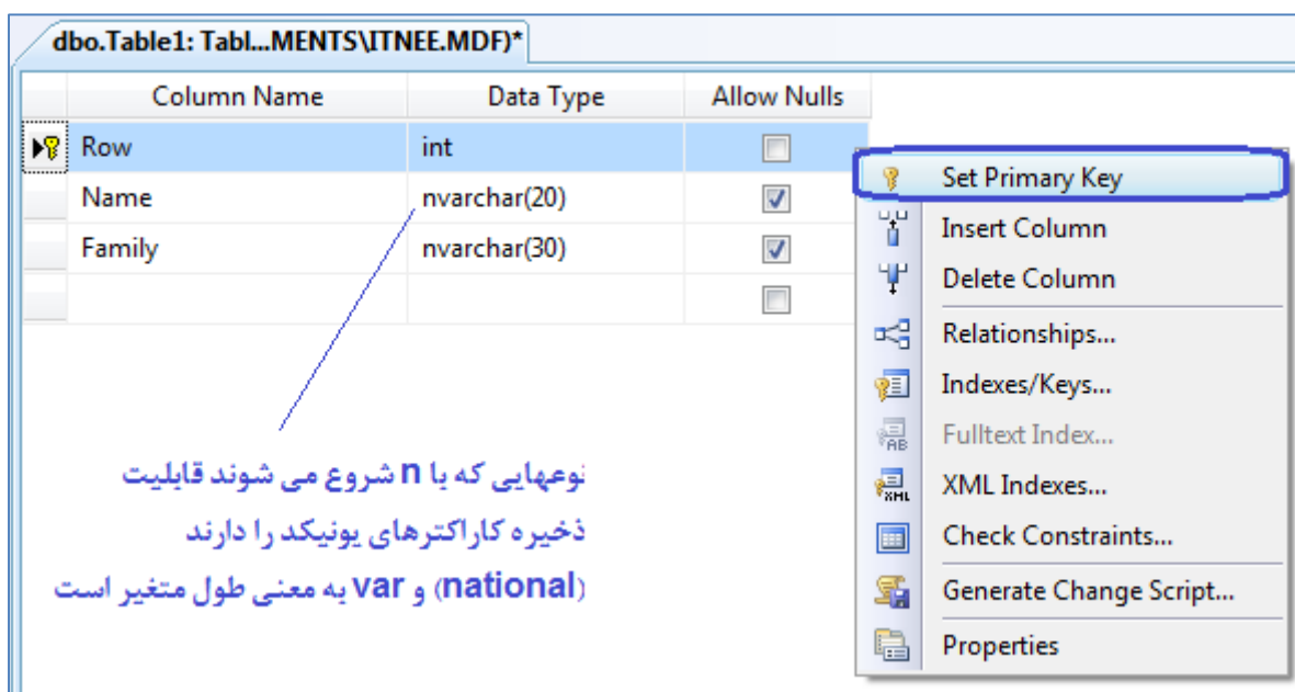
شکل ۶ - جزئیات ایجاد جدول
