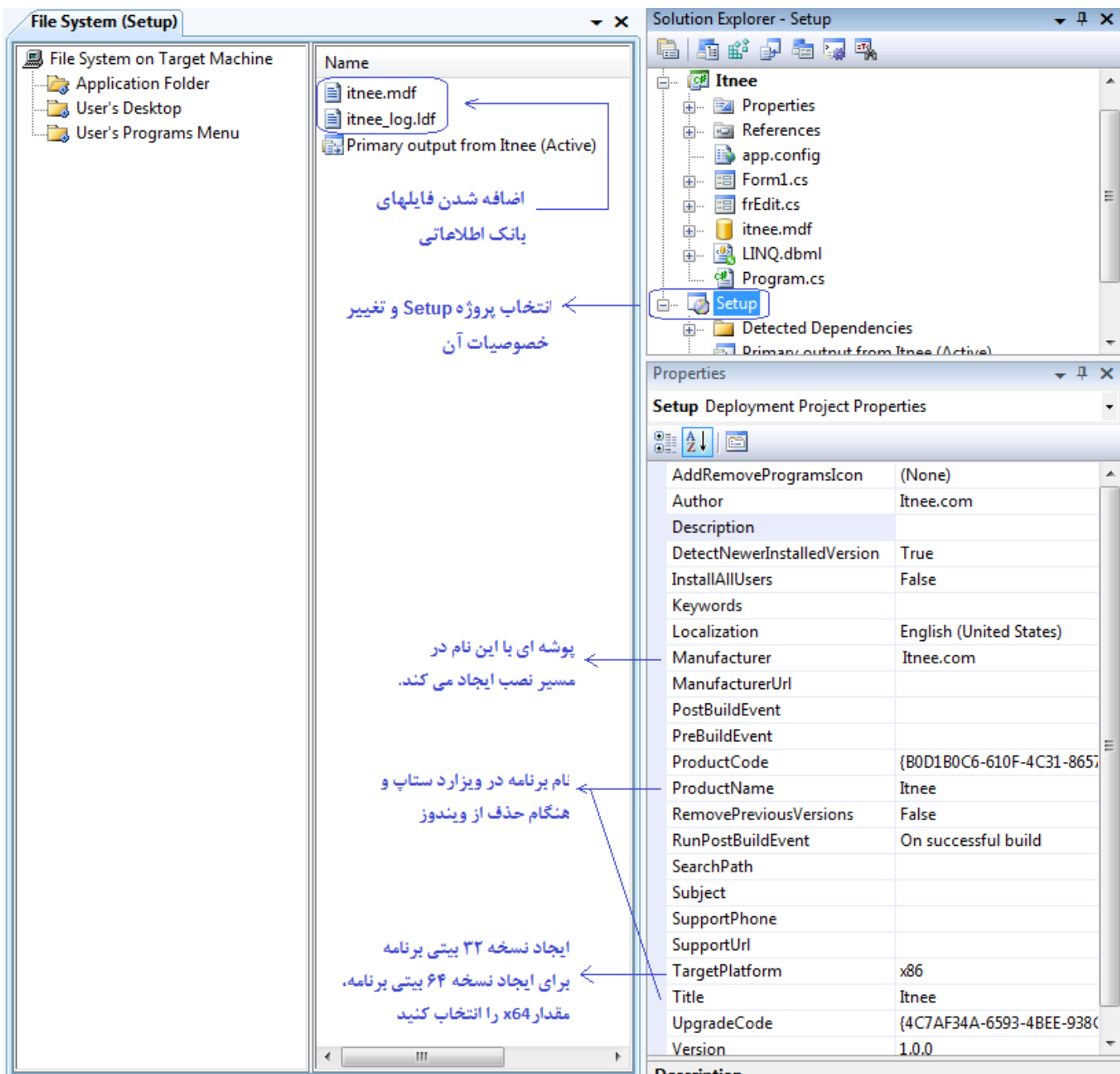
شکل ۲۴ - سفارشی کردن پروژه Setup
