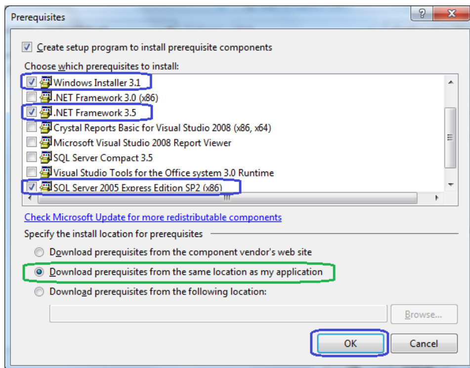
شکل ۲۶ - انتخاب پیش نیازهای نصب برنامه و اضافه کردن آنها به پوشه Setup
