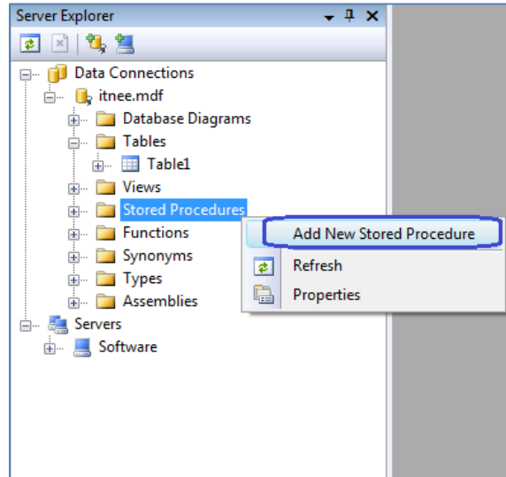
شکل ۸ - ایجاد پروسیجر ذخیره شده برای انجام اعمال ذخیره، ویرایش و حذف از جدول بانک اطلاعاتی
