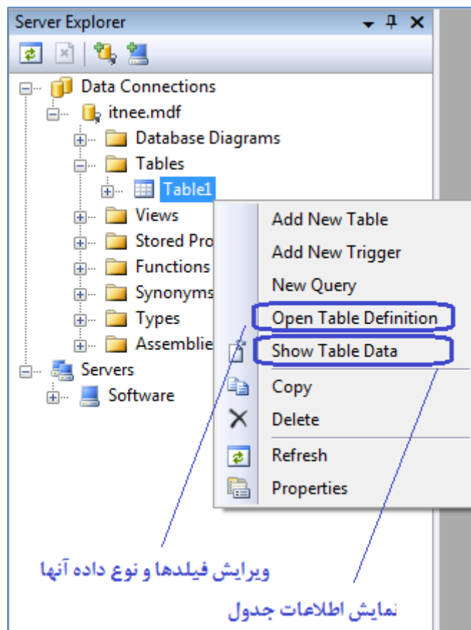
شکل ۷ - انجام تغییرات روی ساختار جدول و یا نمایش داده های آن
