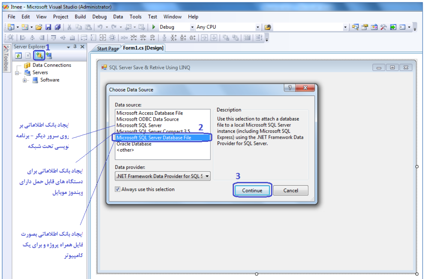
شکل ۲- انتخاب نوع بانک اطلاعاتی
